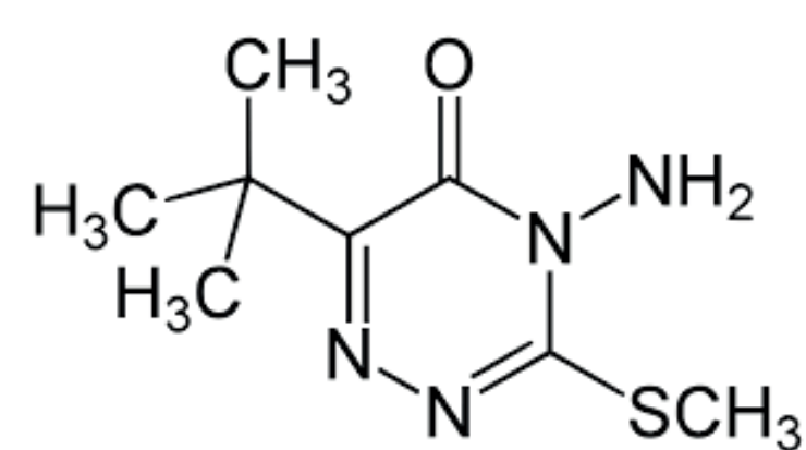
Metribuzin
