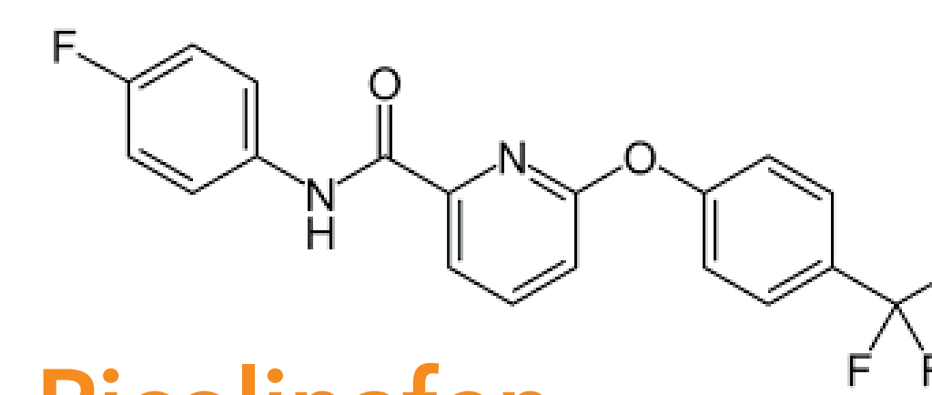
Picolinafen
