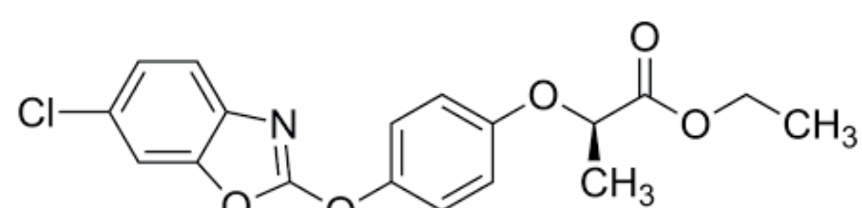
Fenoxaprop-ethyl
