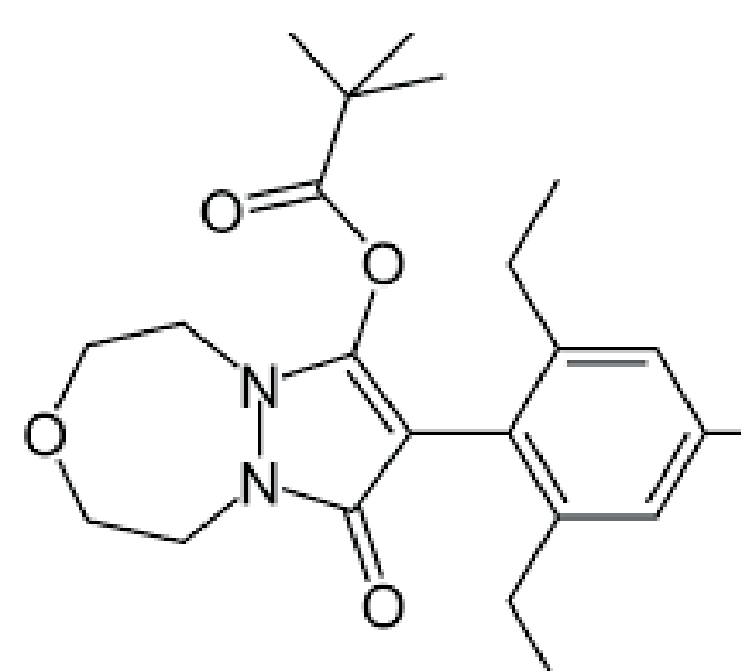
Pinoxaden
