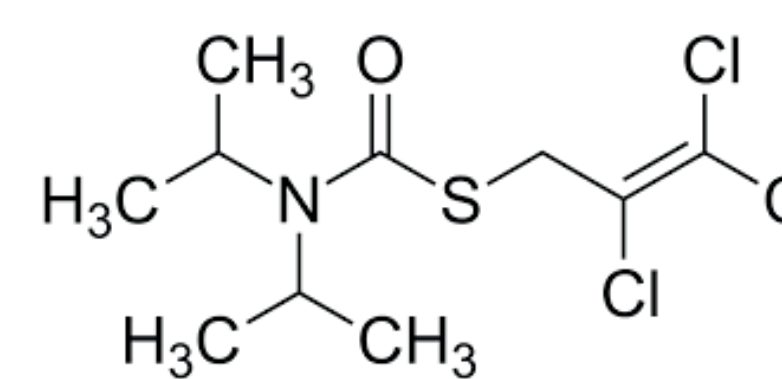
Tri-allate
