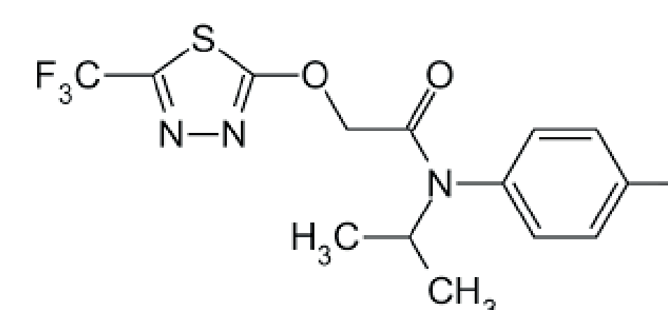
Flufenacet
