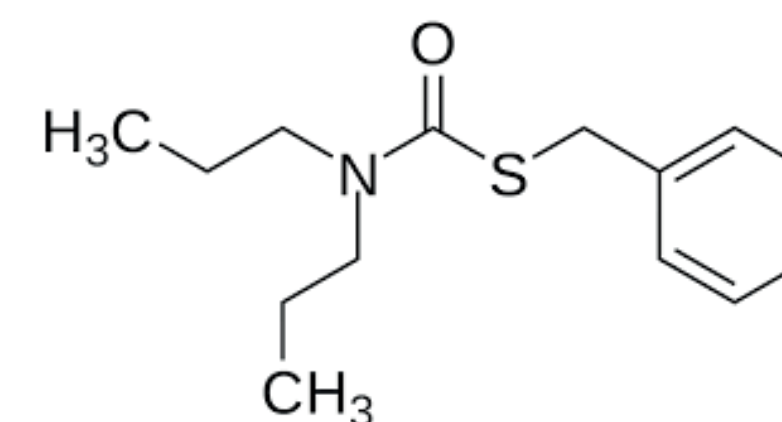
Prosulfocarb
