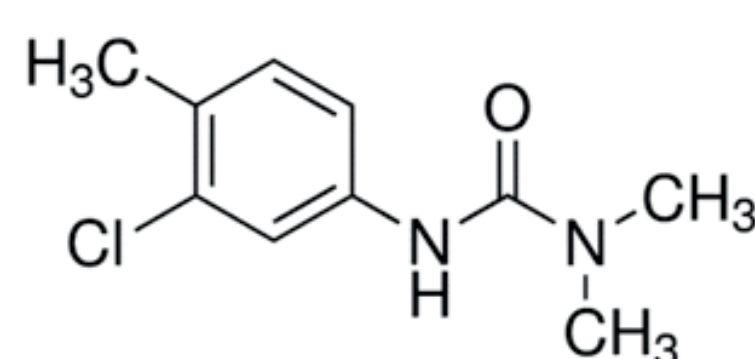
Chlorotoluron
